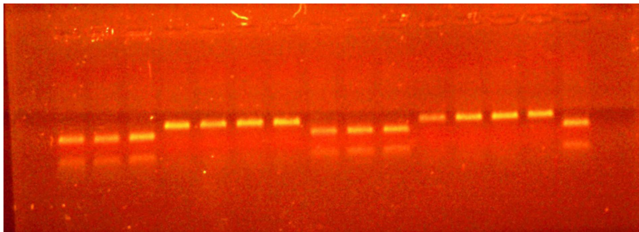
Figura 2. Perfil molecular del marcador CAPS sobre el gen Rrs2.
